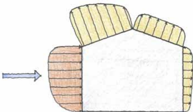
Figur 3 Tryckbild kring en byggnad orsakad av vind.
